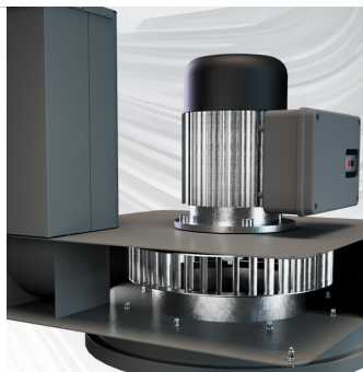
MOTORIZZAZIONE Ventilatore centrifugo da 2,2 KW
